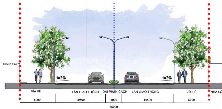
Hình 1. Mặt cắt tuyến trục chính
