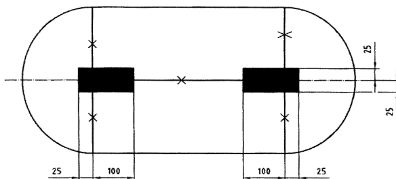
Hình 10 – Kích thước chụp ảnh tia bức xạ các mối hàn – Chai có mối hàn theo chu vi và mối hàn dọc
