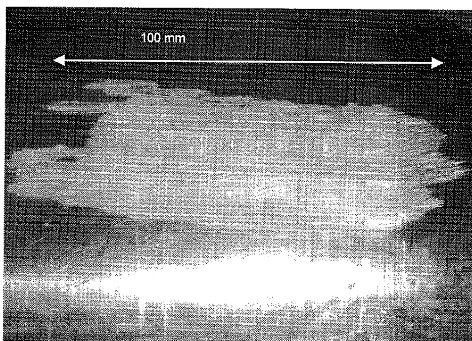
Hình 1. Hư hỏng do cháy xước
