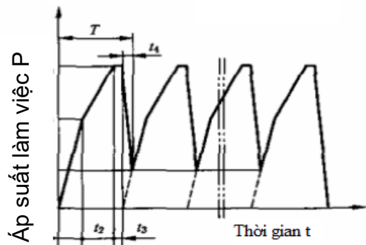
Hình 26. Chu kỳ đặt tải
