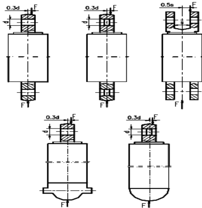
Hình 28. Đặt tải lệch tâm kích chống
