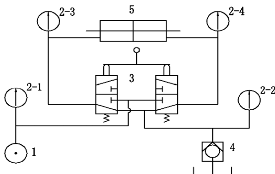
Hình 34. Sơ đồ nguyên lý thử nghiệm khả năng đổi hướng của van đổi hướng
