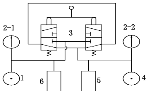
Hình 36: Sơ đồ nguyên lý thử nghiệm an toàn của van khi bị dội áp suất trở lại trở lại của van đổi hướng
