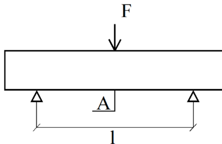
Hình 2. Sơ đồ thử nghiệm gia tải xà
