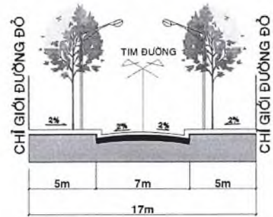
MẶT CẮT 4-4
