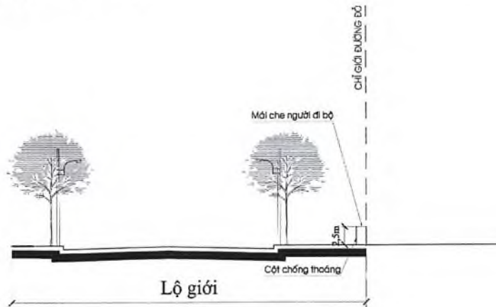
Hình 14 Tường rào xây dựng tạm cho dự án đang xây dựng
