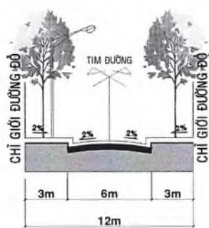
MẶT CẮT 7-7
