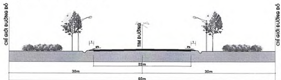
MẶT CẮT 2-2 QUỐC LỘ 1
