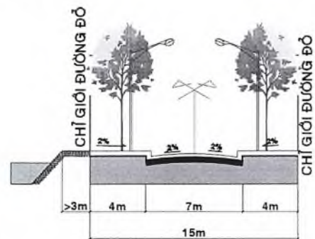
MẶT CẮT 6-6
