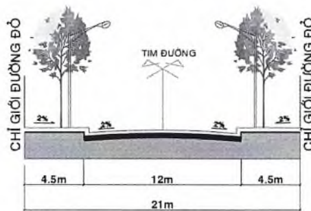
MẶT CẮT 3-3
