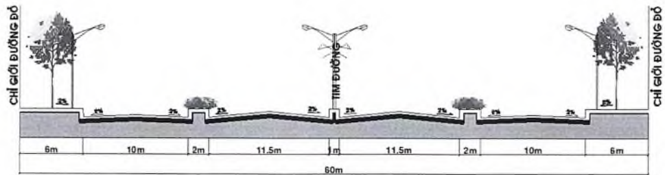
MẶT CẮT 1-1 QUỐC LỘ 1
