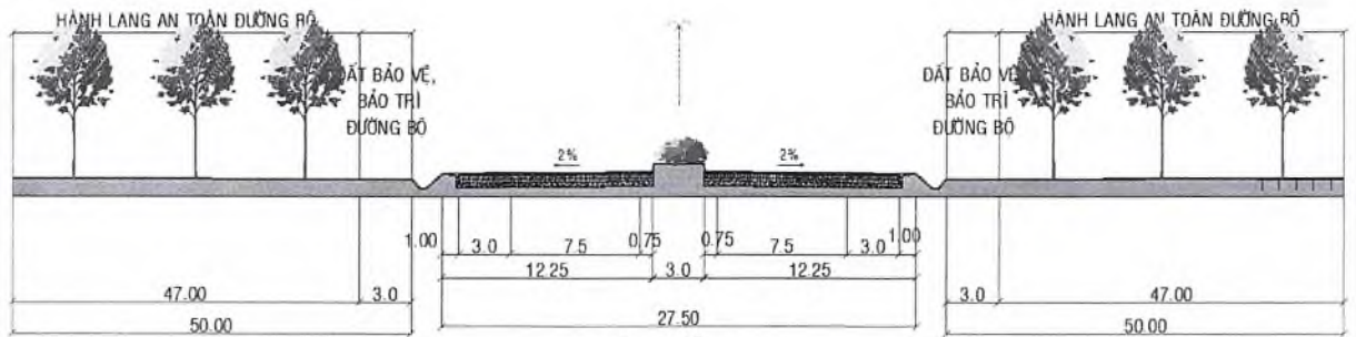
MẶT CẮT A-A ĐƯỜNG CAO TỐC TP. HỒ CHÍ MINH - CẦN THƠ
