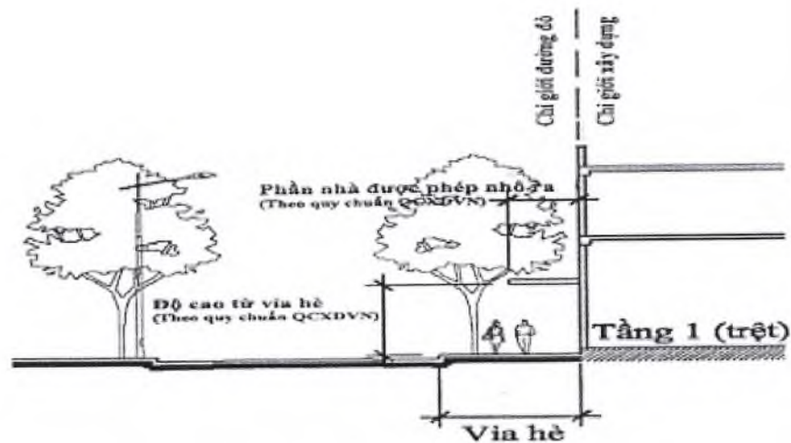
Hình 15 Hình minh họa mái đón, mái hè phố
