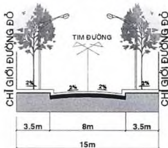
MẶT CẮT 5-5
