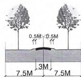
ĐƯỜNG LIÊN ẤP (CẤP A) MẶT CẮT 8-8
