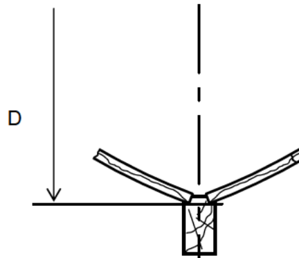
Hình 2 Chiều cao mạn lý thuyết (D) tàu vỏ gỗ
