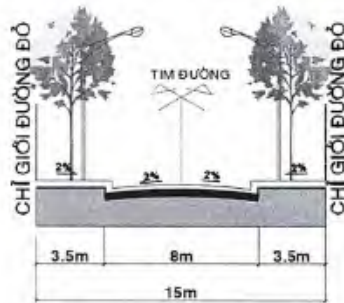
MẶT CẮT 5-5
