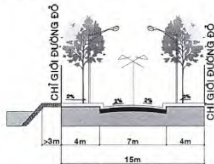
MẶT CẮT 6-6
