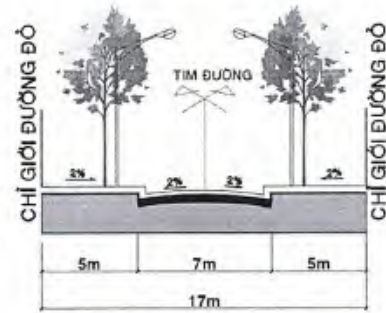
MẶT CẮT 4-4
