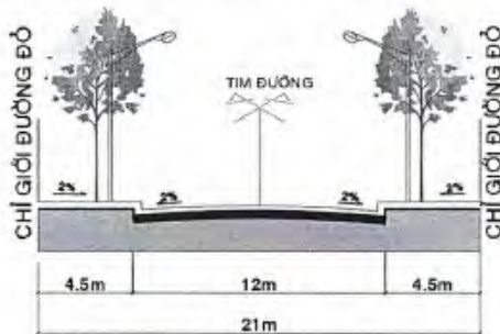
MẶT CẮT 3-3
