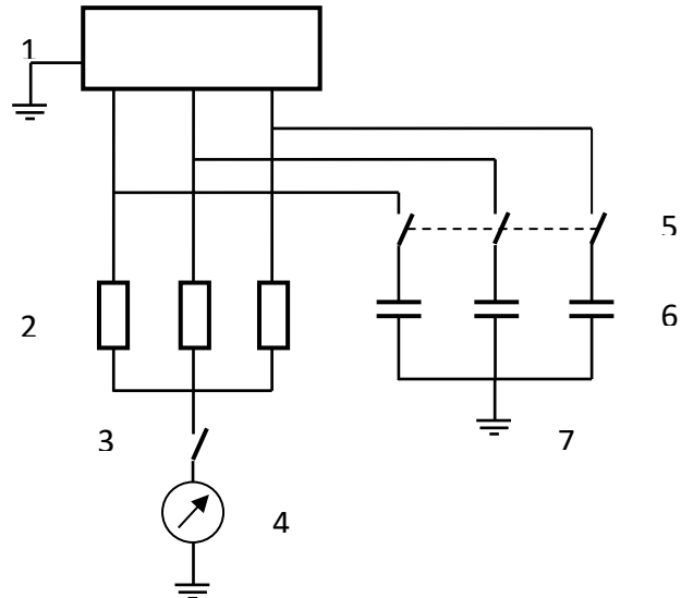
Hình 10. Sơ đồ mô phỏng thử nghiệm rò 3 pha đối xứng
