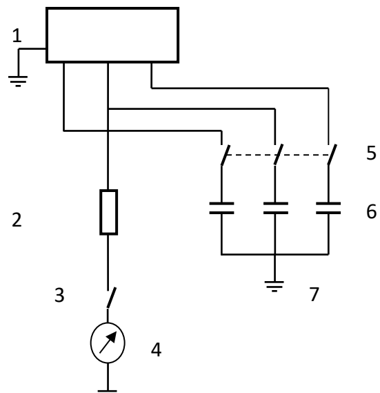
Hình 11. Sơ đồ mô phỏng thử nghiệm rò điện 1 pha
