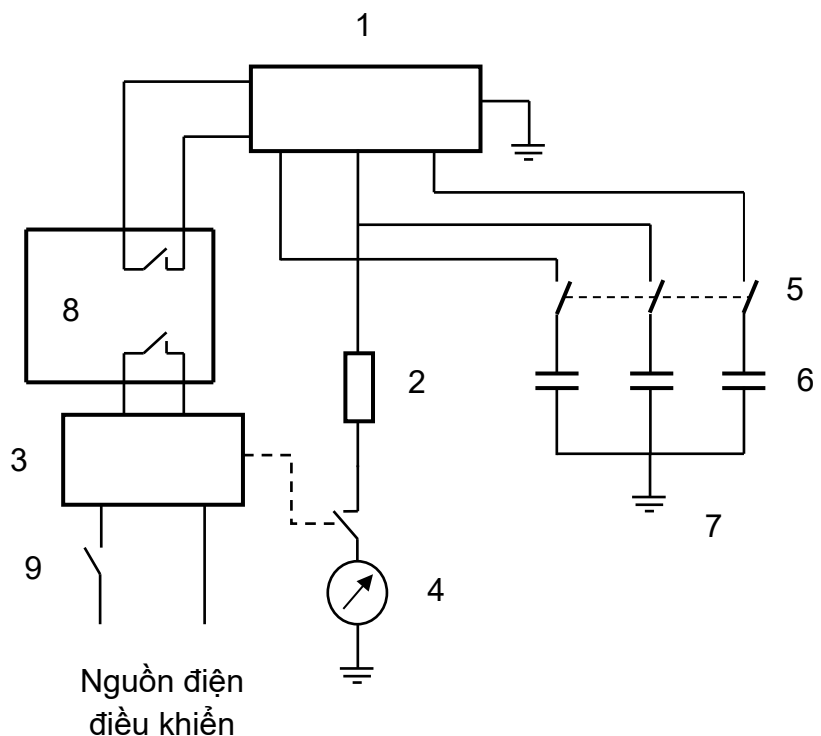
Hình 12. Sơ đồ mô phỏng xác định thời gian cắt khi rò điện 1k \Omega
