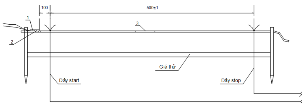
Hình 1 - Sơ đồ đấu nối dây nổ thường để đo tốc độ nổ
