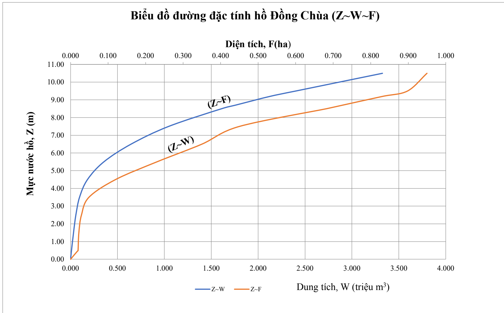
Hình II-3: Biểu đồ quan hệ mực nước, dung tích, diện tích mặt hồ
