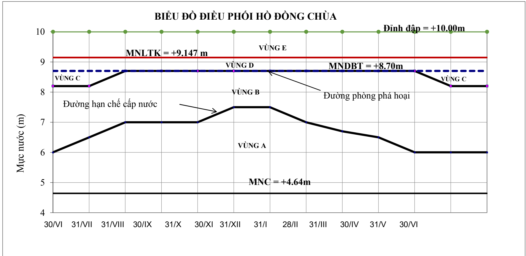
Hình II-2: Biểu đồ điều phối hồ chứa nước
