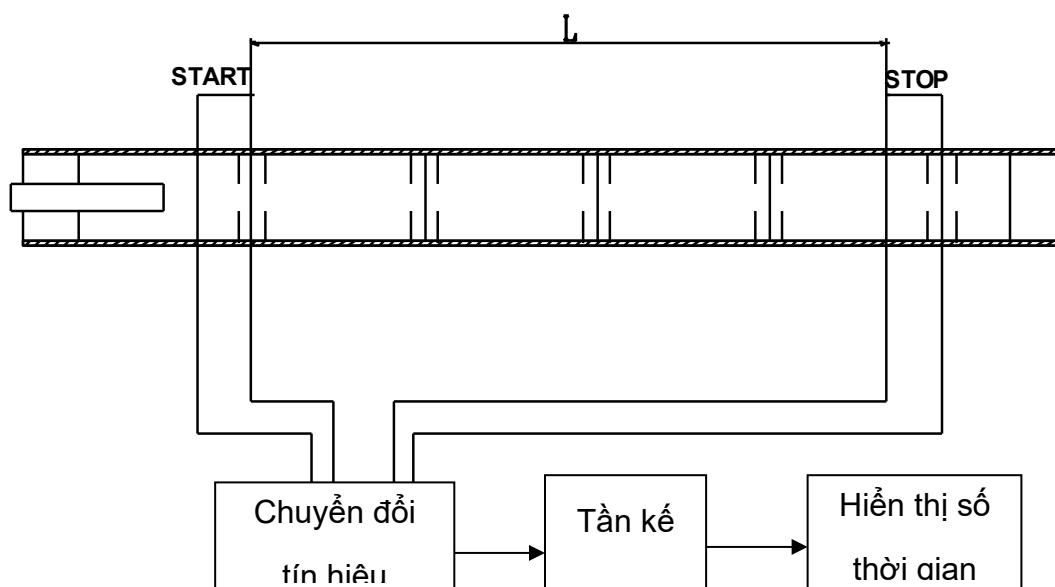
Hình 6. Sơ đồ đầu nối và chuẩn bị đo tốc độ nổ
