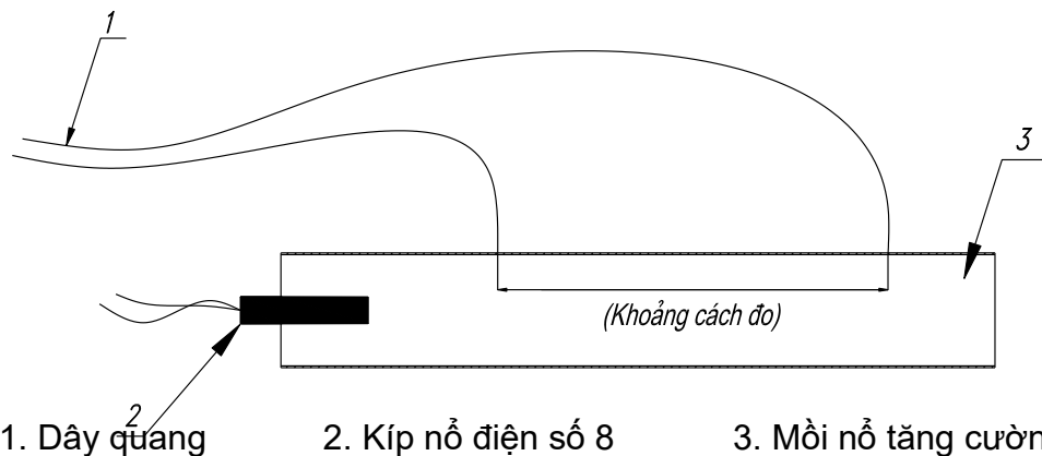
Hình 2. Sơ đồ chuẩn bị mẫu và cách đấu dây với mẫu mồi nổ tăng cường
