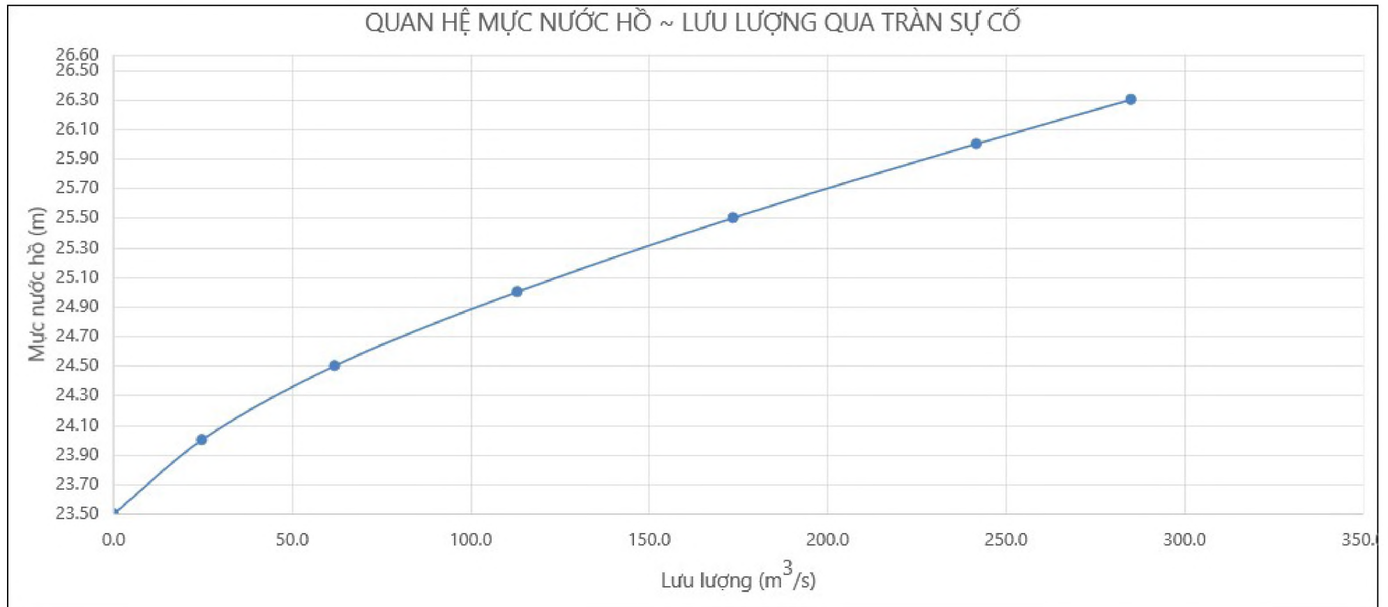
Hình PL 5.5: Lưu lượng qua tràn ~ Mực nước hồ (Tràn sự cố)
