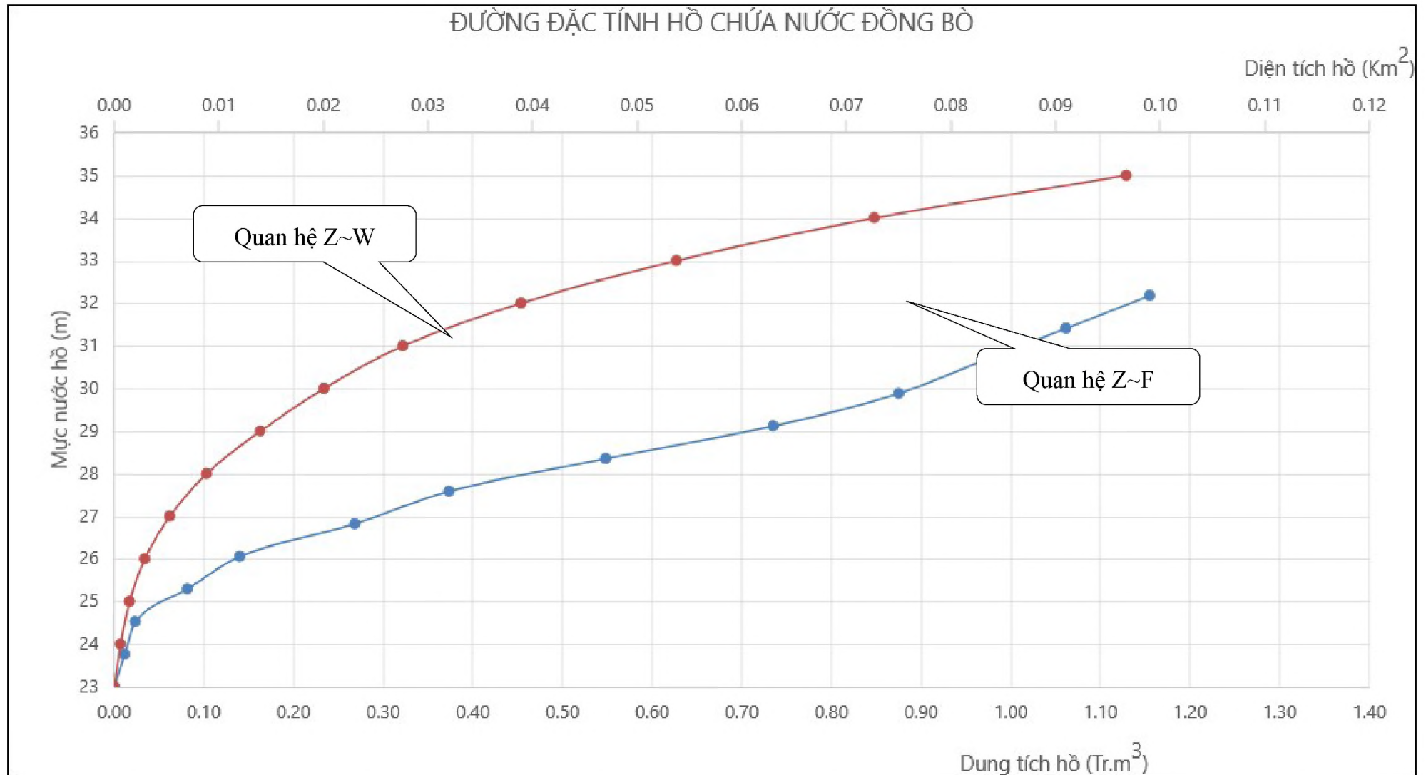
Hình PL8.1 Đường đặc tính hồ chứa nước Đồng Bò
