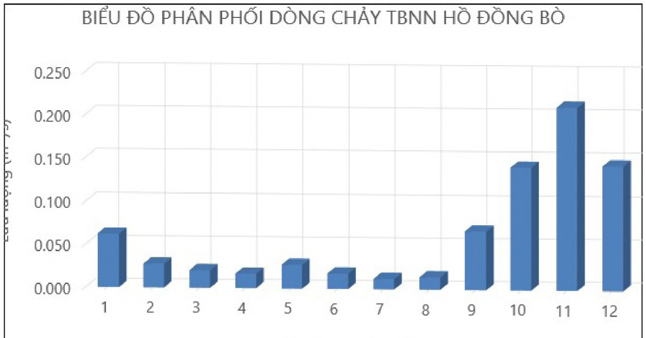
Hình PL 2.1 : Hình vẽ biểu đồ dòng chảy TBNN đến hồ Đồng Bò
