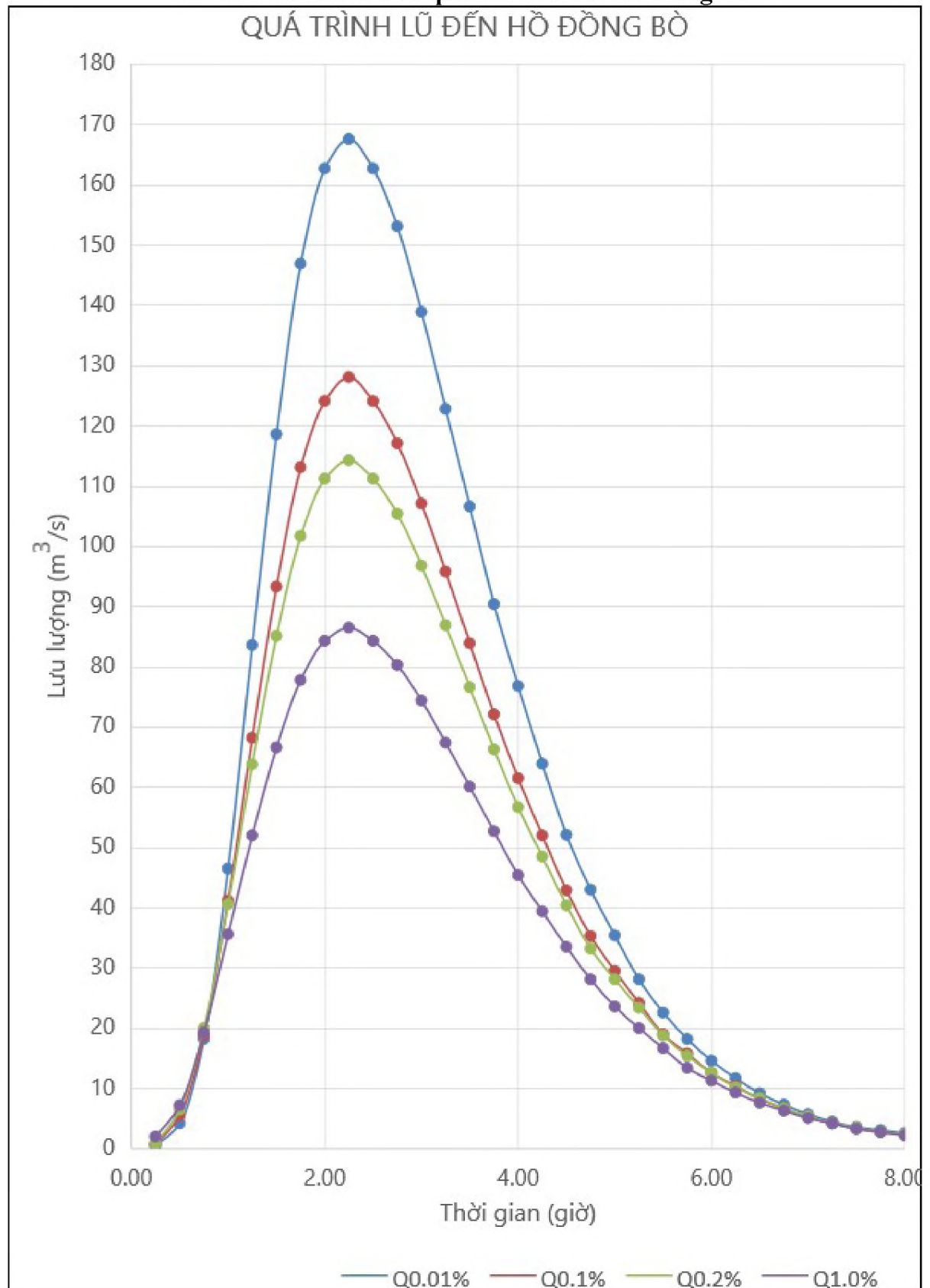
Hình PL 2.2 : Hình vẽ quá trình lũ đến hồ Đồng Bò
