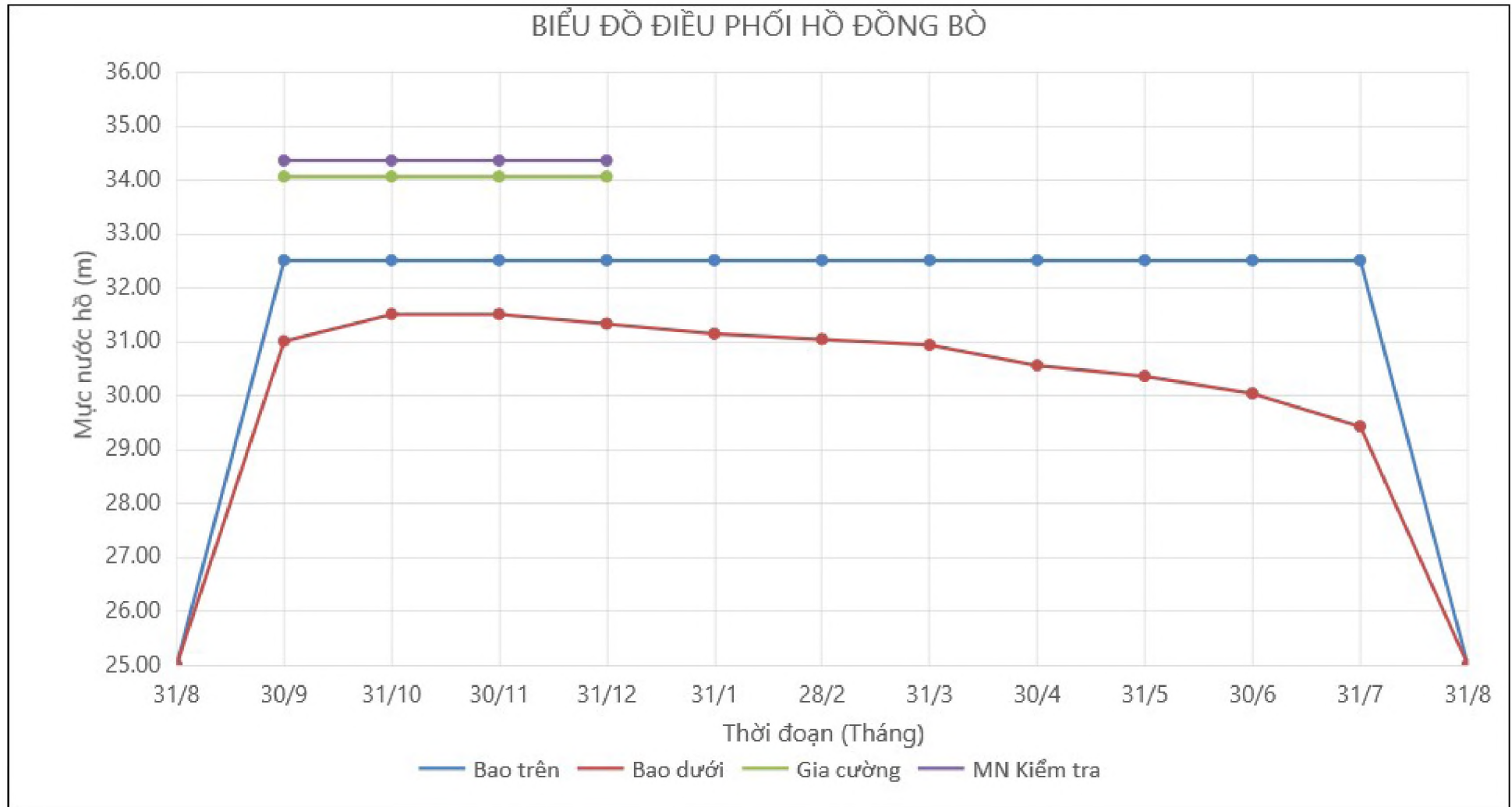
Hình PL7.1 Biểu đồ điều phối hồ chứa nước Đồng Bò
