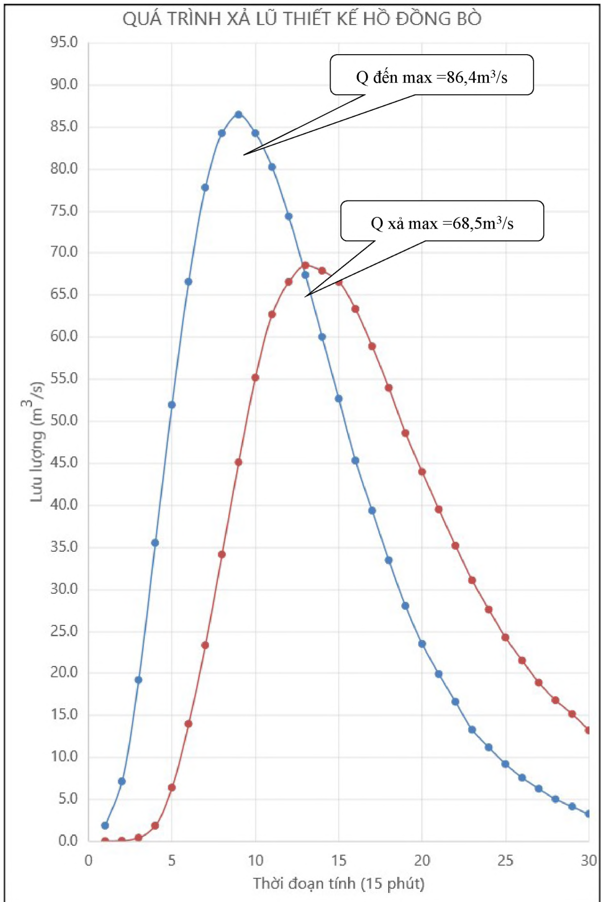
Hình PL 4.1: Quá trình điều tiết lũ thiết kế
