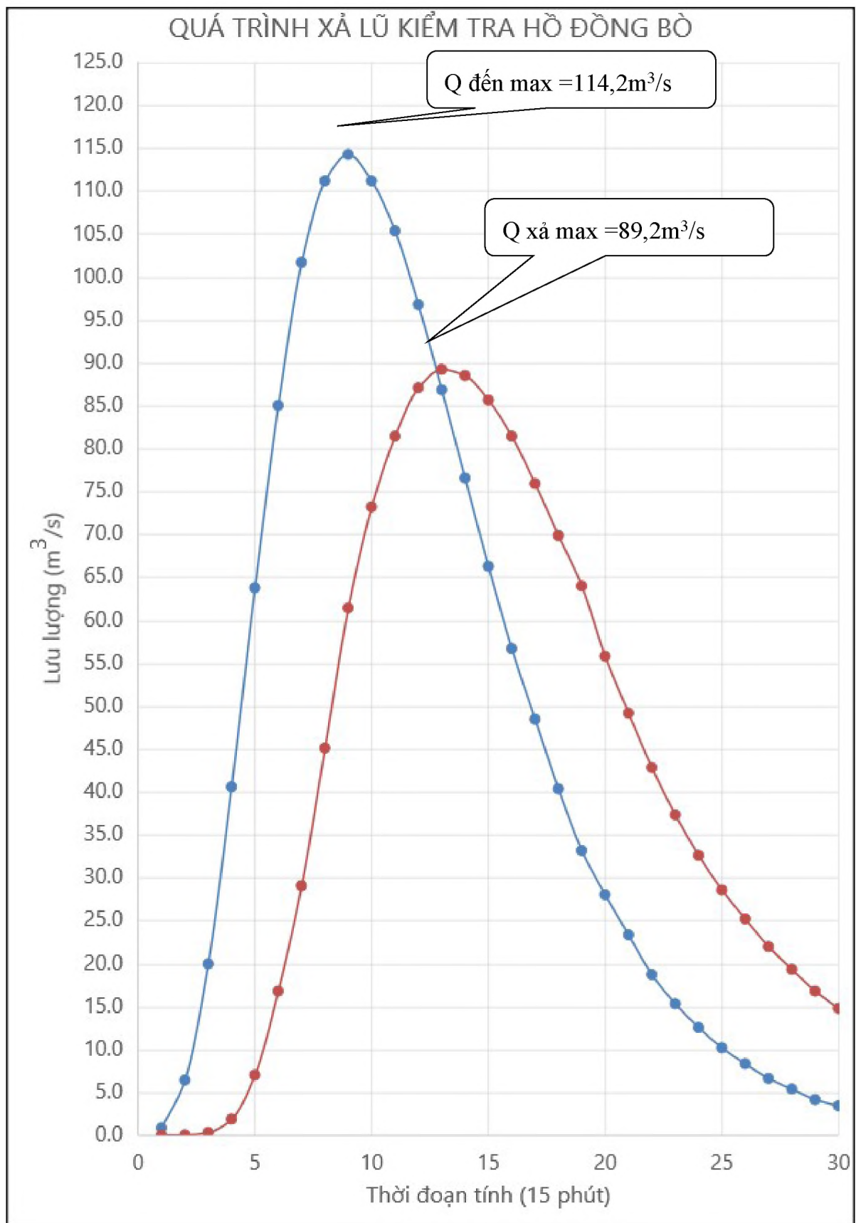
Hình PL 4.2: Quá trình điều tiết lũ kiểm tra
