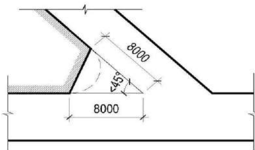
Vát góc tại góc cắt giao lộ nhỏ hơn 45^0
