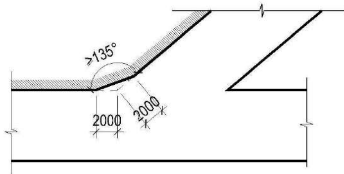
Kích thước vát góc tại góc cắt giao lộ lớn hơn 135^0
