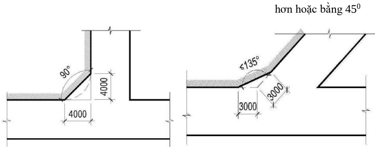
Kích thước vát góc tại góc cắt giao với lộ giới bằng 90^0
